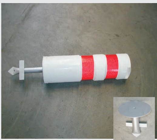
Balisette mit Stahlanker (feuerverzinkt) zur Befestigung im Bankett / Soft bollard with galvanised steel anchor (installation in shoulder)
