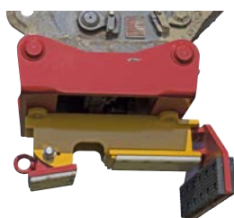
Verbaugreifer
